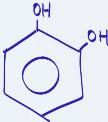
रेसॉरिनॉल
