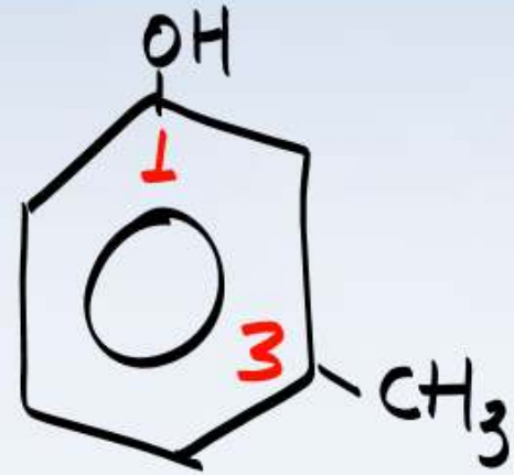
m - क्रीसॉल
