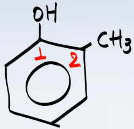
o - क्रीसॉल
