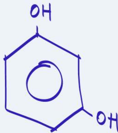
रेसॉरिनॉल
