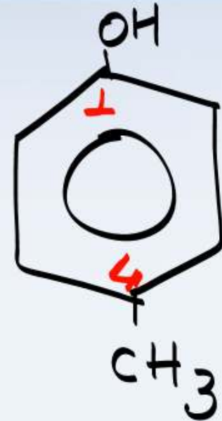
p - क्रीसॉल
